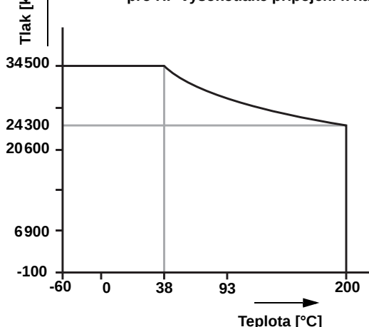
Graf závislosti procesního tlaku na procesní teplotě pro HP vysokotlaké připojení k nádrži
