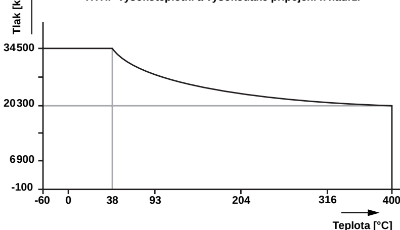
Graf závislosti procesního tlaku na procesní teplotě pro HTHP vysokoteplotní a vysokotlaké připojení k nádrži
