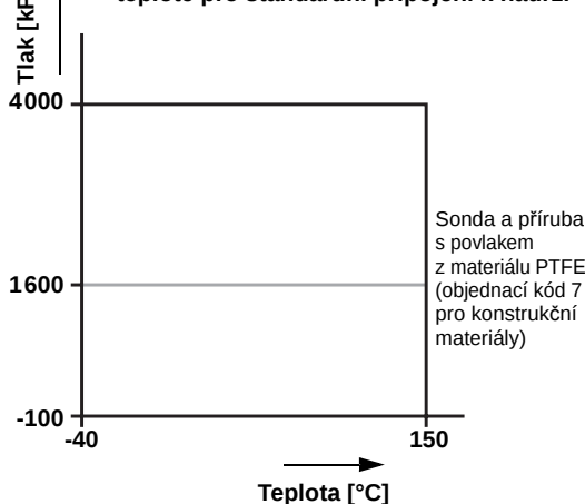
Graf závislosti procesního tlaku na procesní teplotě pro standardní připojení k nádrži
