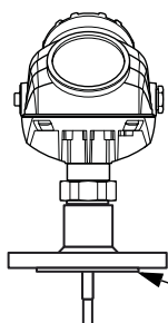
Konstrukce těsnění nádrže s oddělovací ochrannou deskou
